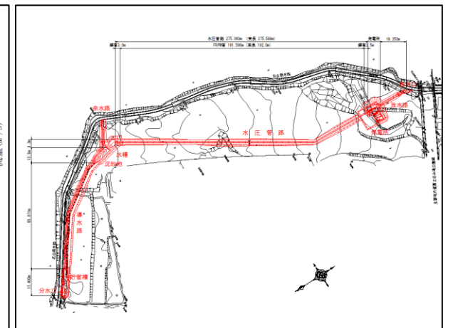
H28 基本設計平面図
