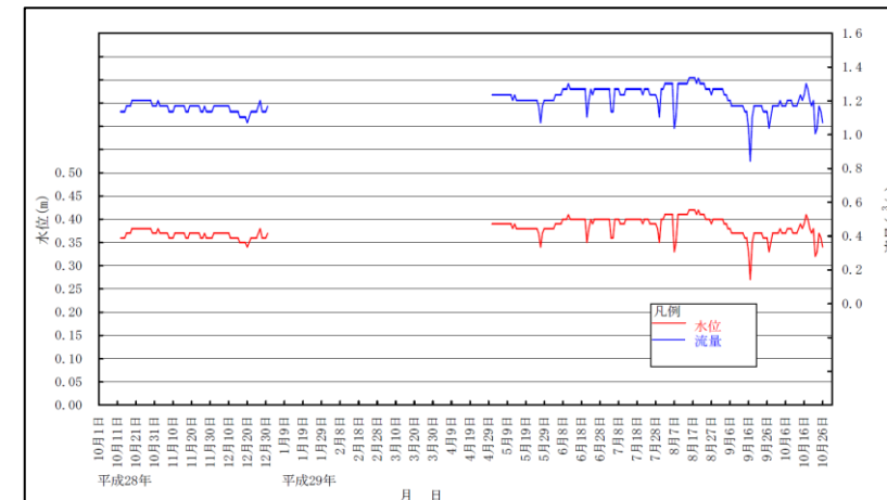
H28~29 年度流量調査結果
