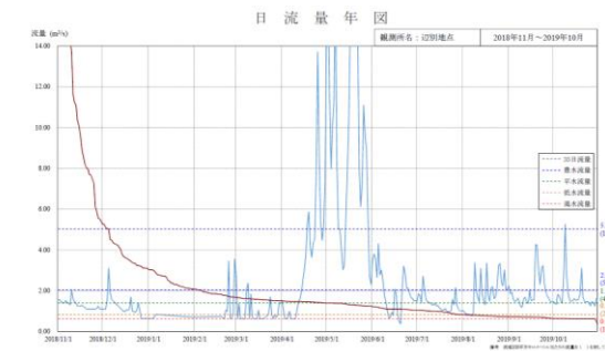
流況表 (流量及び水位)
